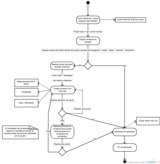
Figura 4: Esquema de Ecuador científico.
