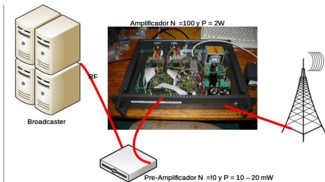
Figura 1. Esquema de los equipos de transmisión.
