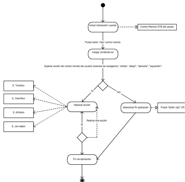
Figura 1: Esquema general de la aplicación interactiva “programa Miradas”
