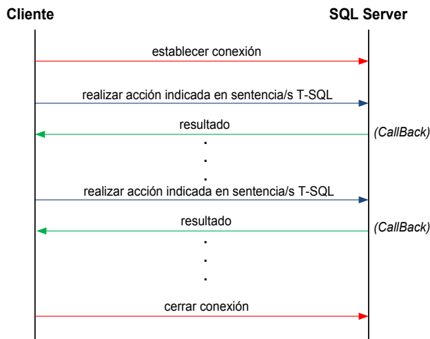
Figura 3. Procedimiento de comunicación con SQL Server.
