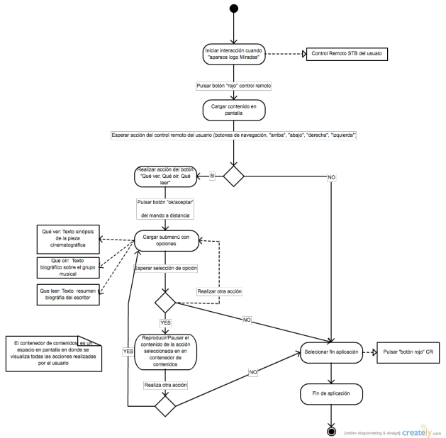
Figura 7: Esquema de entretenimiento.
