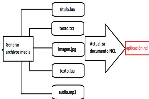
Figura 5. Actualización de documento NCL.
