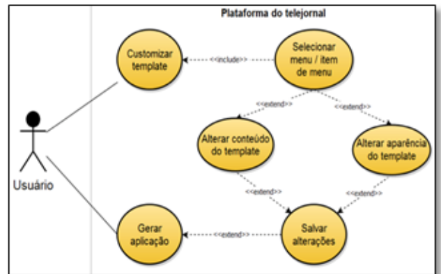
Figure 2: Requisitos funcionais da plataforma
